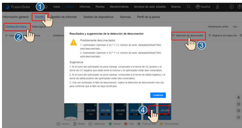
Figura 3-4 Detección de desconexión de los optimizadores
