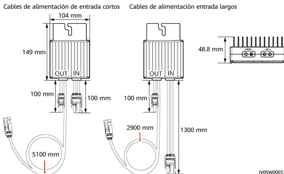
Figura 2-3 Dimensiones del optimizador
