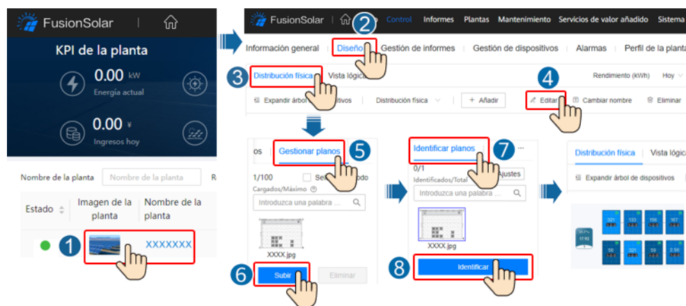
Figura 3-1 Diseño de distribución física de módulos FV
