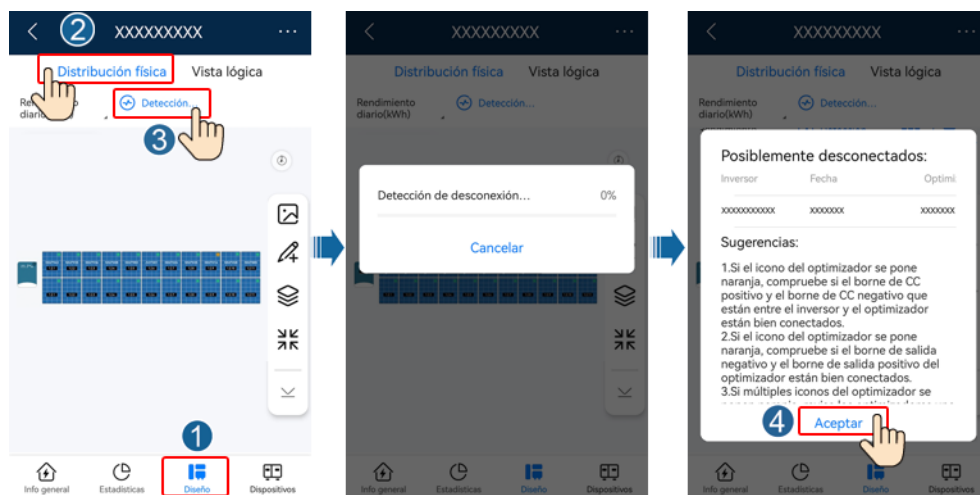
Figura 3-3 Detección de desconexión de los optimizadores
