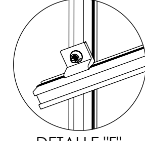
DETALLE "F" NXT-CRC Conexión de Tensor
