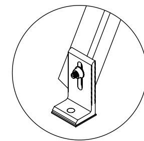
DETALLE "D" NXT-LFOOT Conector de riel RX
