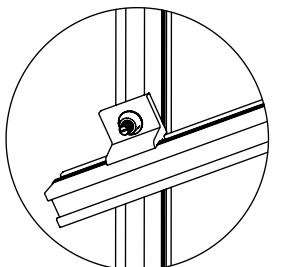
DETALLE "F" NXT-CRC Conexión de Tensor
