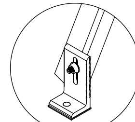
DETALLE "D" NXT-LFOOT Conector de riel RX
