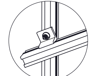
DETALLE "F" NXT-CRC Conexión de Tensor
