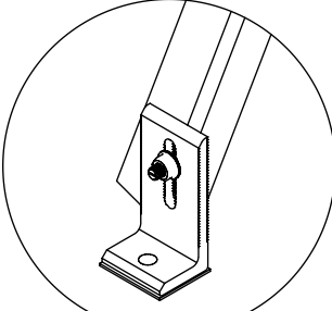
DETALLE "E" NXT-LFOOT Conector de riel RX
