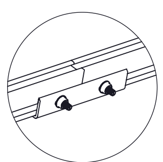
DETALLE "C" NXT-RS Empalme de riel RX
