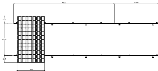
VISTA PLANTA
