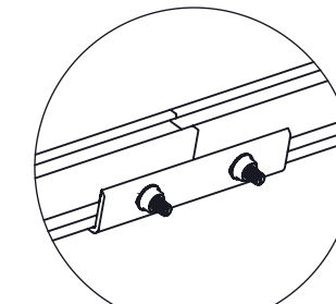
DETALLE "C" NXT-RS Empalme de riel RX
