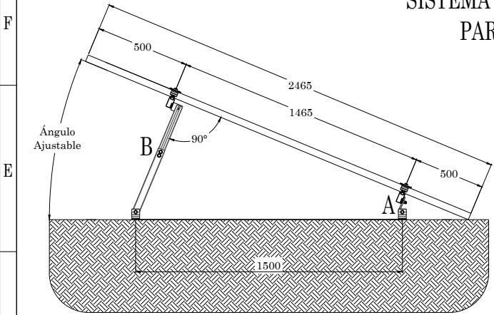
VISTA LATERAL
