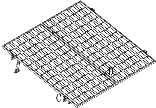
VISTA ISOMÉTRICA
