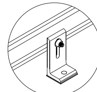
DETALLE "C" NXT-LFOOT Soporte de riel RX
