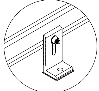
DETALLE "C" NXT-LFOOT Soporte de riel RX
