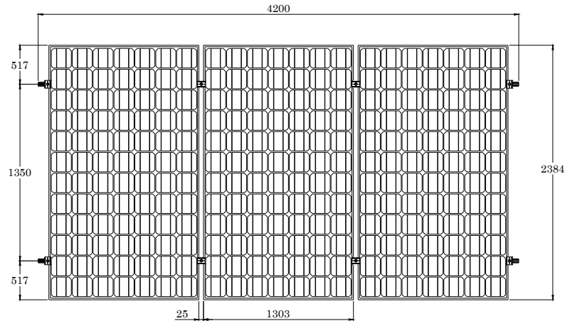
VISTA PLANTA
