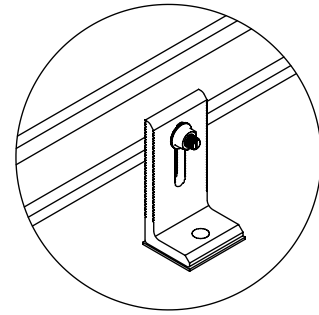
DETALLE "C" NXT-LFOOT Soporte de riel RX
