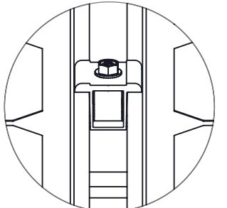
DETALLE "B" NXT-AUA Abrazadera Universal (Modo Intermedio)
