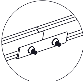
DETALLE "G" NXT-RS Empalme de riel RX
