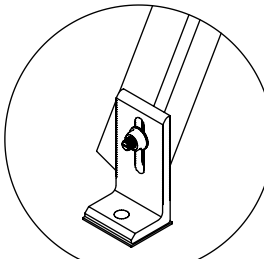
DETALLE "E" NXT-LFOOT Conector de riel RX
