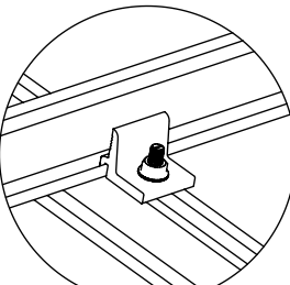
DETALLE "C" NXT-CRC Clip de Conexión Transversal
