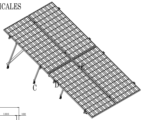
VISTA ISOMÉTRICA
