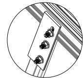
DETALLE A Conector Ángulo Riel
