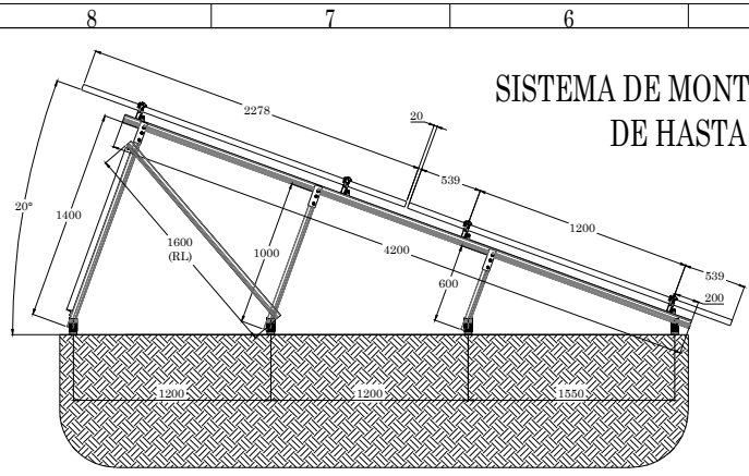
VISTA LATERAL
