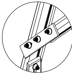
DETALLE "H" Conexión de Tensor
