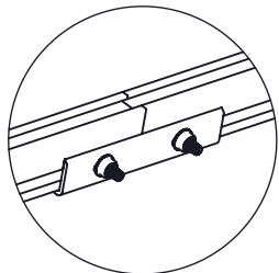
DETALLE "G" NXT-RS Empalme de riel RX
