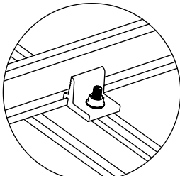
DETALLE "C" NXT-CRC Clip de Conexión Transversal
