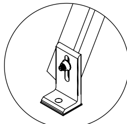
DETALLE "E" NXT-LFOOT Conector de riel RX
