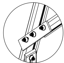
DETALLE "H" Conexión de Tensor
