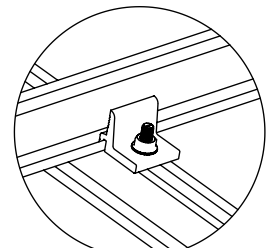
DETALLE "C" NXT-CRC Clip de Conexión Transversal
