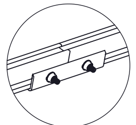
DETALLE "G" NXT-RS Empalme de riel RX
