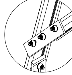
DETALLE "G" Conexión de Tensor
