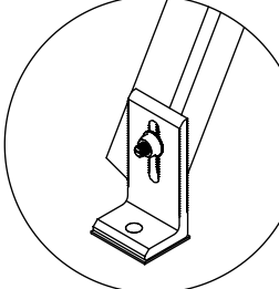
DETALLE "E" NXT-LFOOT Conector de riel RX
