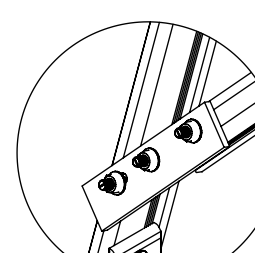
DETALLE "G" Conexión de Tensor
