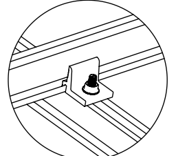
DETALLE "C" NXT-CRC Clip de Conexión Transversal
