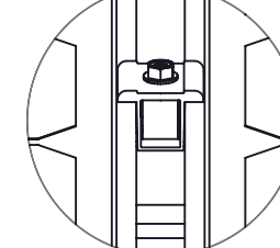
DETALLE "B" NXT-AUA Abrazadera Universal (Modo Intermedio)
