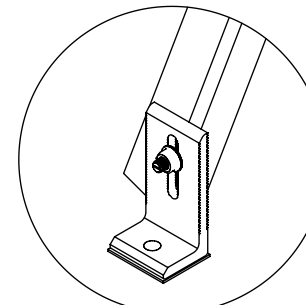
DETALLE "E" NXT-LFOOT Conector de riel RX
