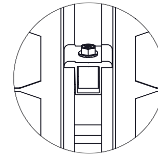
DETALLE "B" NXT-AUA Abrazadera Universal (Modo Intermedio)
