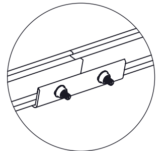
DETALLE "C" NXT-RS Empalme de riel RX
