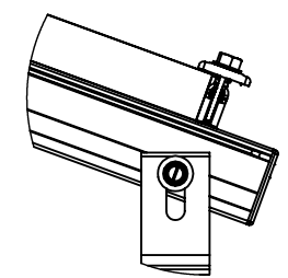
Detalle 4 Cross Clamp Posición Final
