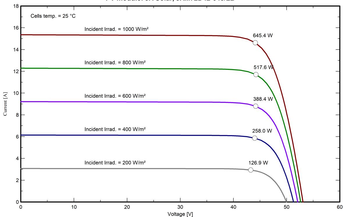
PV module: JA Solar, JAM72D42-645/LB
